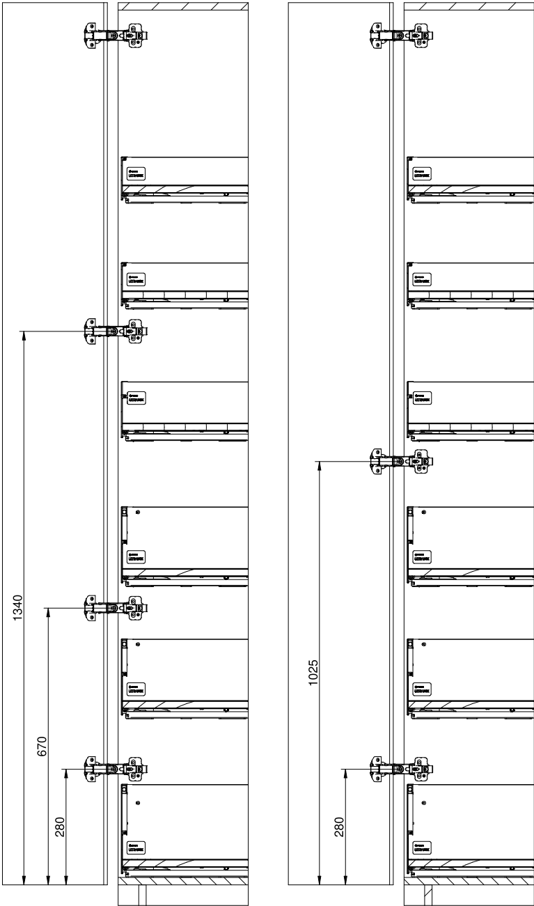
Drilling measurements - front Установка петель - фасад Встановлення петель - фасад
