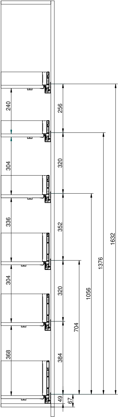
Positioning in the cabinet Разметка установки в корпусе Розташування в корпусі
