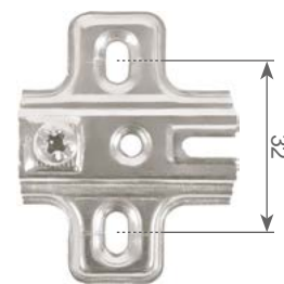
Mounting regulation Возможность регулировки Регуляція на планці
