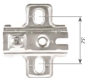
Mounting regulation Возможность регулировки Регуляція на планці
